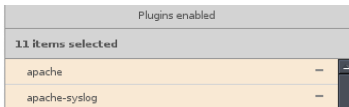
Εικόνα 0-20 Ενεργοποιημένες επεκτάσεις
