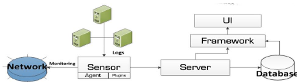
Εικόνα 4-3 OSSIM Sensor
