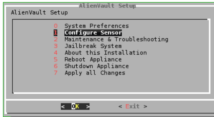
Εικόνα 0-21 Μενού τερματικού
