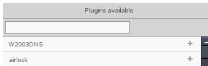
Εικόνα 0-19 Ενεργοποίηση επεκτάσεων
