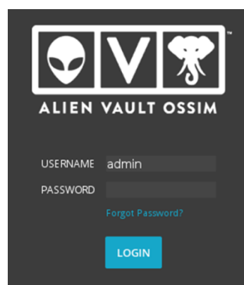
Εικόνα 4-4 User Login
