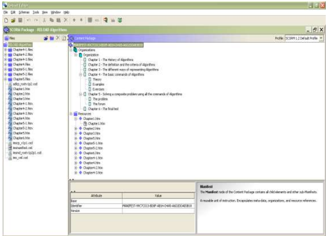
Εικόνα 2.1. Reload Editor
