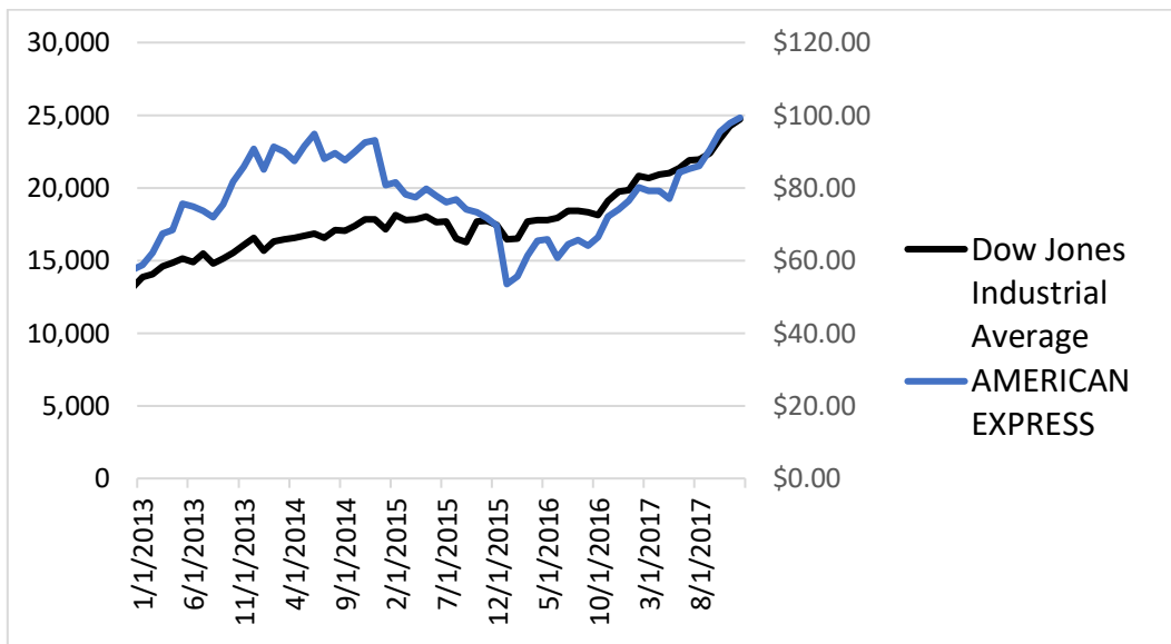
Διάγραμμα 2.2: Η πορεία του Dow Jones Industrial Average και της εταιρείας American Express την περίοδο 31/12/2012 έως 29/12/2017 (Μηνιαία στοιχεία)
