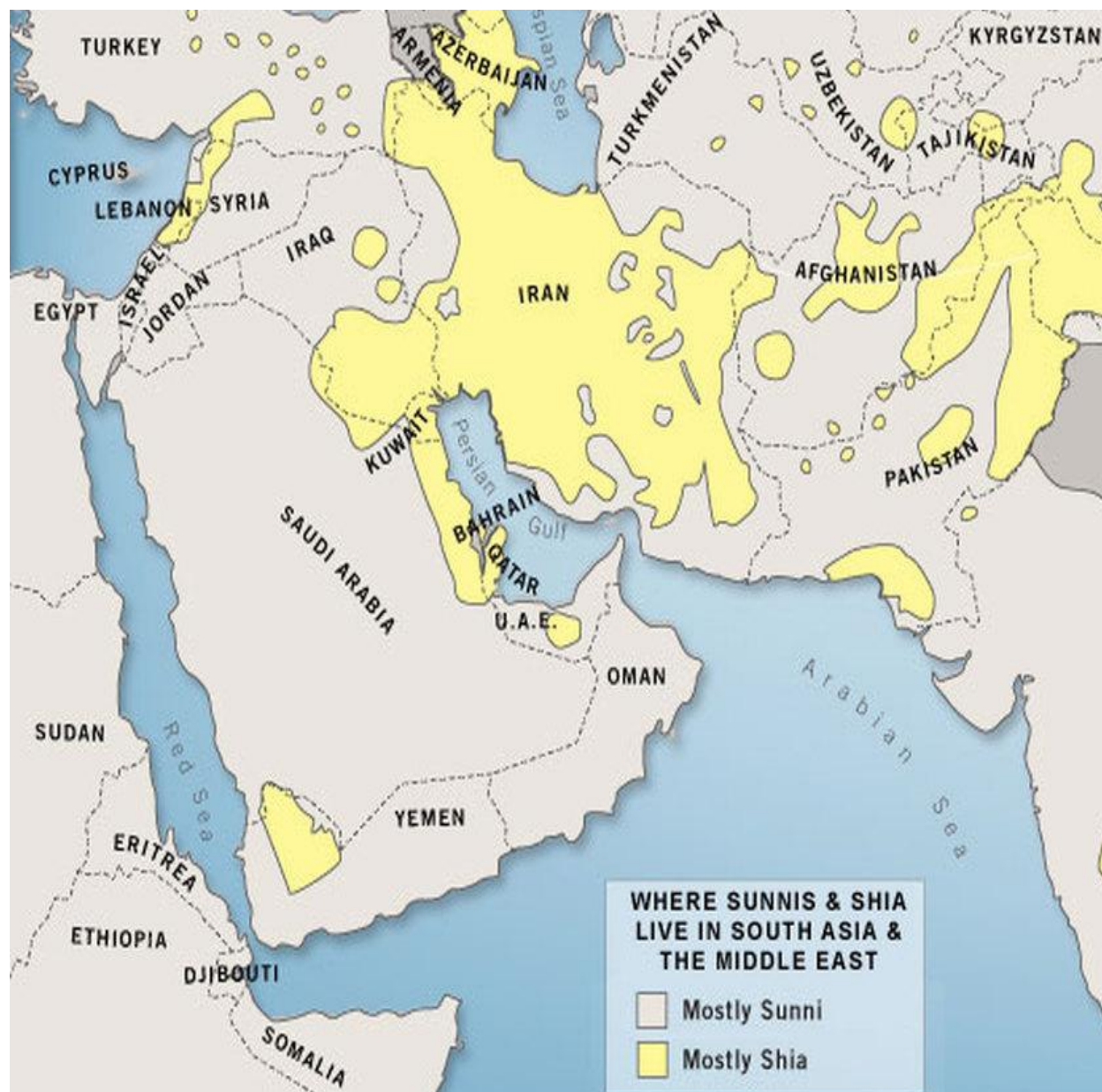
Χάρτης 3: Χάρτης της Μέσης Ανατολής : Σία και Σούννα.
