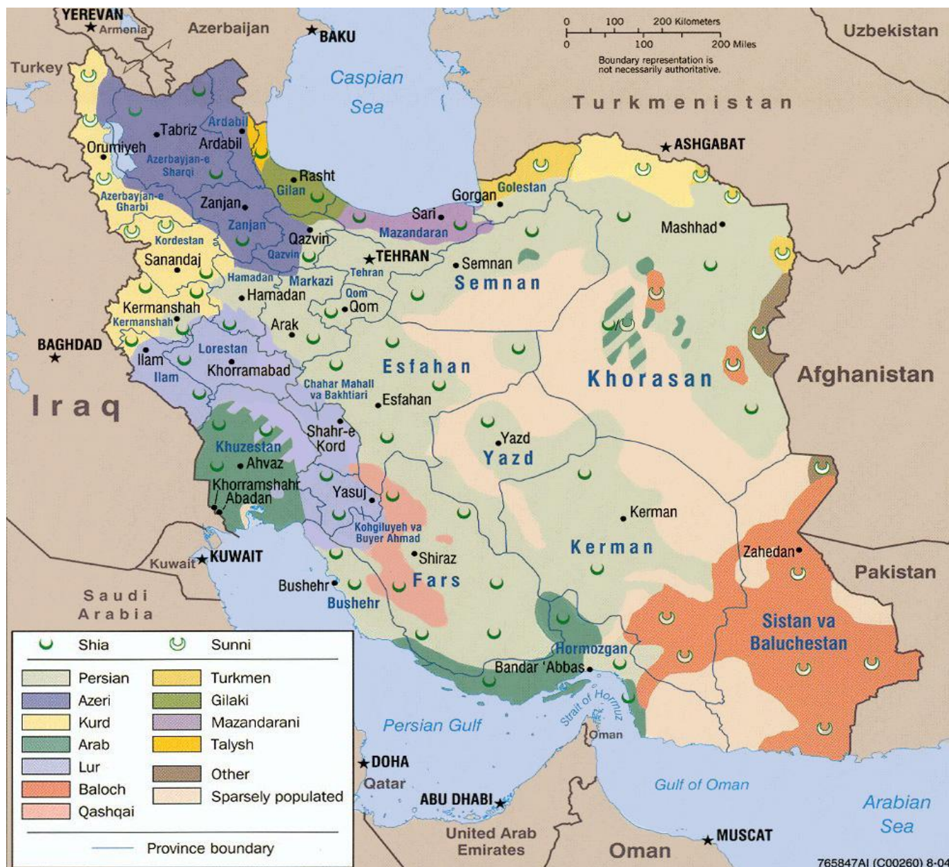
Χάρτης 4: Ο φυλετικός και θρησκευτικός χάρτης του Ιράν.
