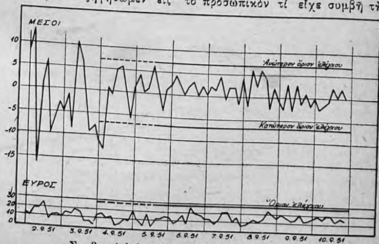
Σχ. 3. Δελτίον έλέγχου έξωτερικής διαμέτρου
