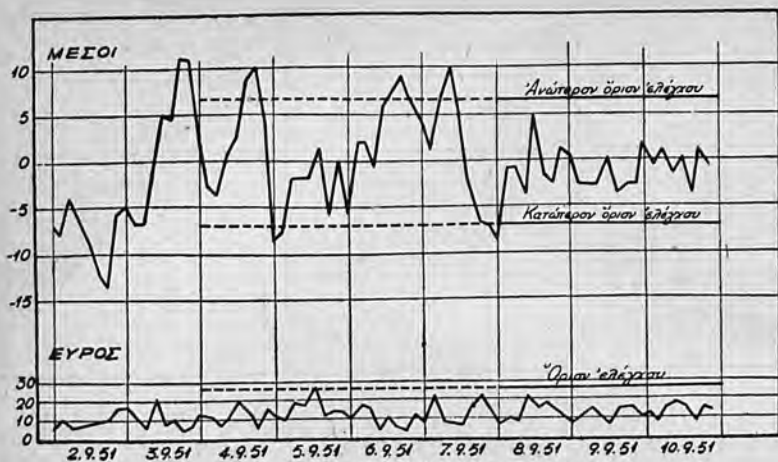
Σχ. 4. Δελτίον έλέγχου έξωτερικής διαμέτρου
