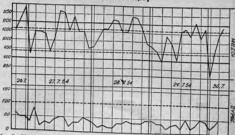
Σχ. 5. Χυτήριο—Έλεγχος της πίεσεως με έκτοξευτήρα άμμου καθαρισμού (παροχή)
