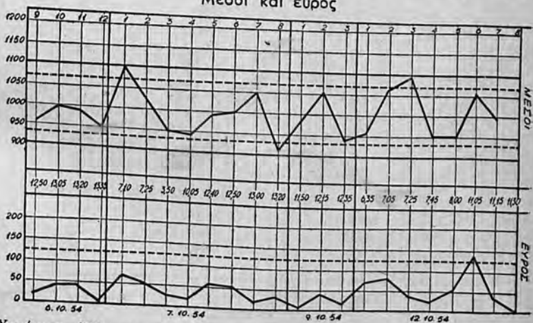
Χυτήριο—Έλεγχος της πίεσεως με έκτοξευτήρα άμμου καθαρισμού (Μετά τον έλεγχον)
