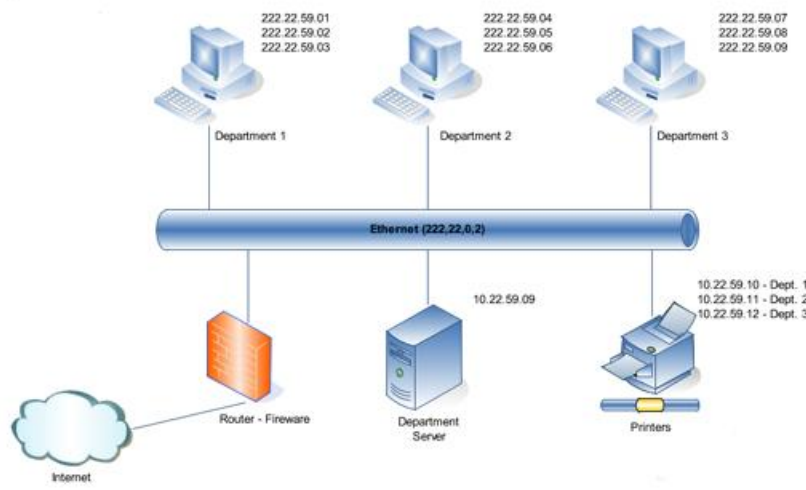
Σχήμα 2: Τοπικό δίκτυο LAN.
