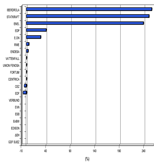
ΠΑΡΑΓΩΓΗ ΕΚΤΟΣ ΣΥΝΟΡΩΝ (2006)
