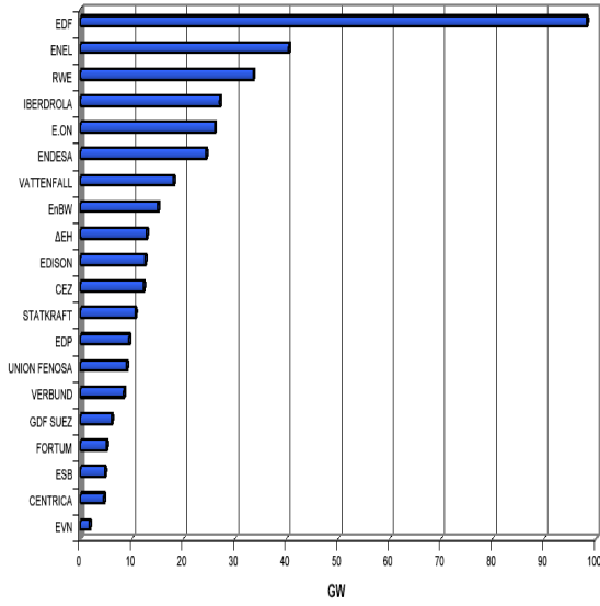
ΕΓΧΩΡΙΑ ΕΓΚΑΤΕΣΤΗΜΕΝΗ ΙΣΧΥΣ (2007)
