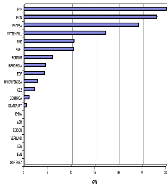
ΕΓΚΑΤΕΣΤΗΜΕΝΗ ΙΣΧΥΣ ΕΚΤΟΣ ΣΥΝΟΡΩΝ (2006)
