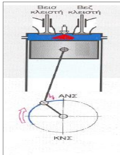
Εικόνα 2.6 Ισόχωρη προσθήκη θερμότητας(OTTO-cycle)
