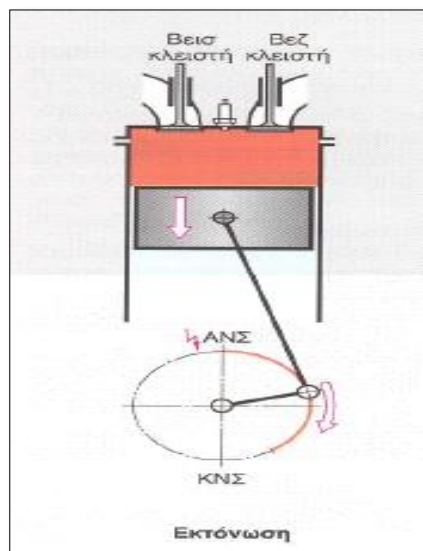
Εικόνα 2.7 Ισεντροπική εκτόνωση-power stroke(OTTO-cycle)
