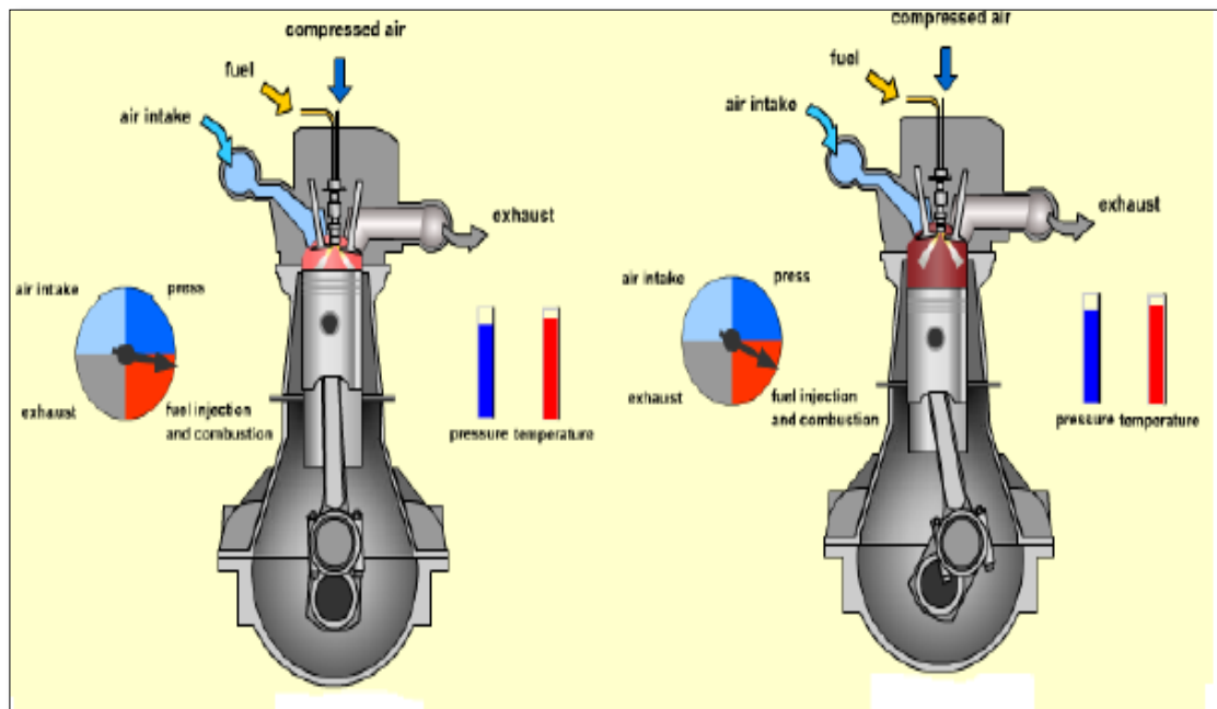
Εικόνα 2.13 Ισοβαρής προσθήκη θερμότητας (DIESEL-cycle).
