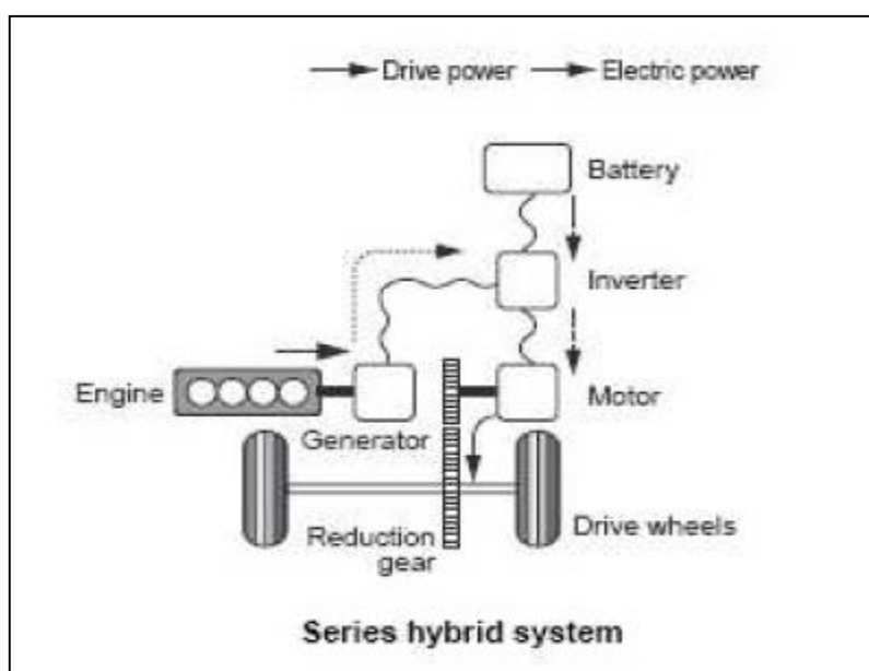
Εικόνα 2.19 Σειριακή διάταξη υβριδικού οχήματος.
