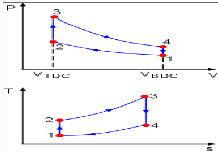
Εικόνα 2.10 Διάγραμμα T-s και P-V ιδανικού κύκλου OTTO
