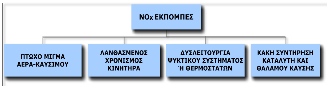
Εικόνα 3.2 Κυριότερες αιτίες εκπομπών NO x από Μ.Ε.Κ.
