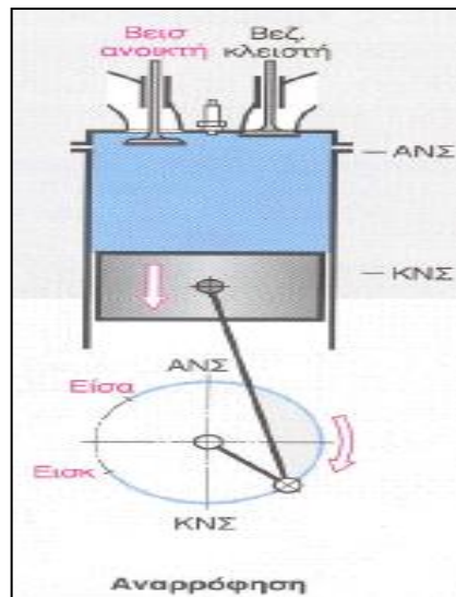
Εικόνα 2.4 Εισαγωγή καυσίμου μίγματος στον θάλαμο καύσης (OTTO-cycle).
