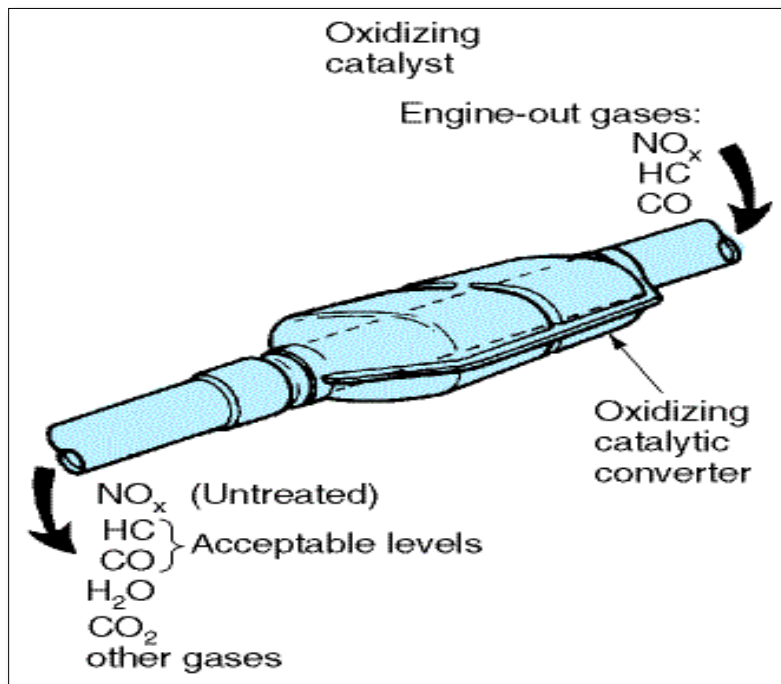
Εικόνα 3.7 Καταλυτικός μετατροπείας οξειδωσης με τα προϊόντα εισόδου και την έξοδό τους
