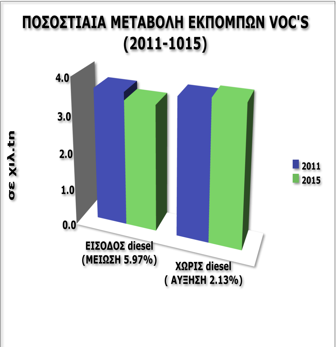
Εικόνα 6.13 Ποσοστιαία μεταβολή εκπομπών VOC'S κατά την διάρκεια εφαρμογής του σεναρίου (2011-2015)
