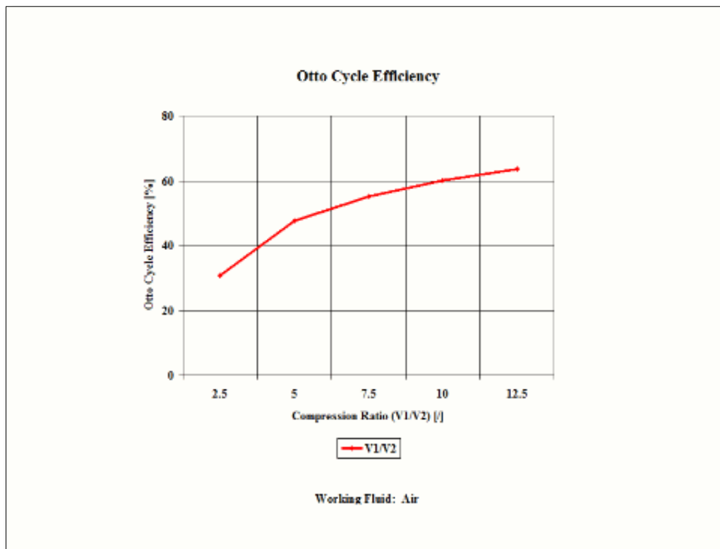
Εικόνα 2.11 Διαγραμματική απεικόνιση συσχέτισης βαθμού απόδοσης με τον λόγο συμπίεσης (κύκλος ΟΤΤΟ)
