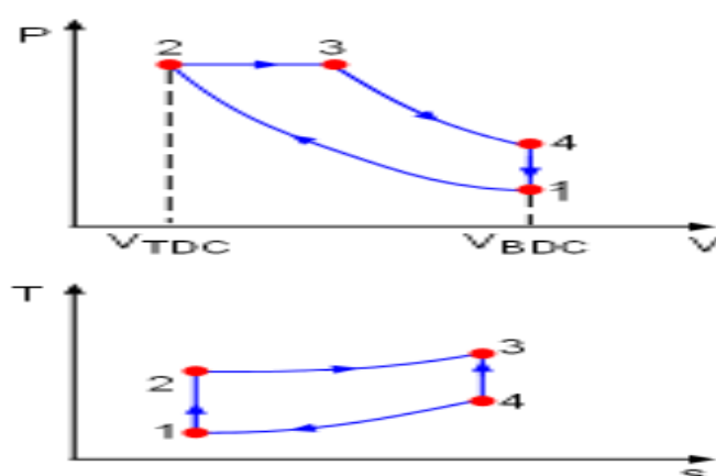
Εικόνα 2.16 Διαγράμματα T-s και P-V ιδανικού κύκλου DIESEL.
