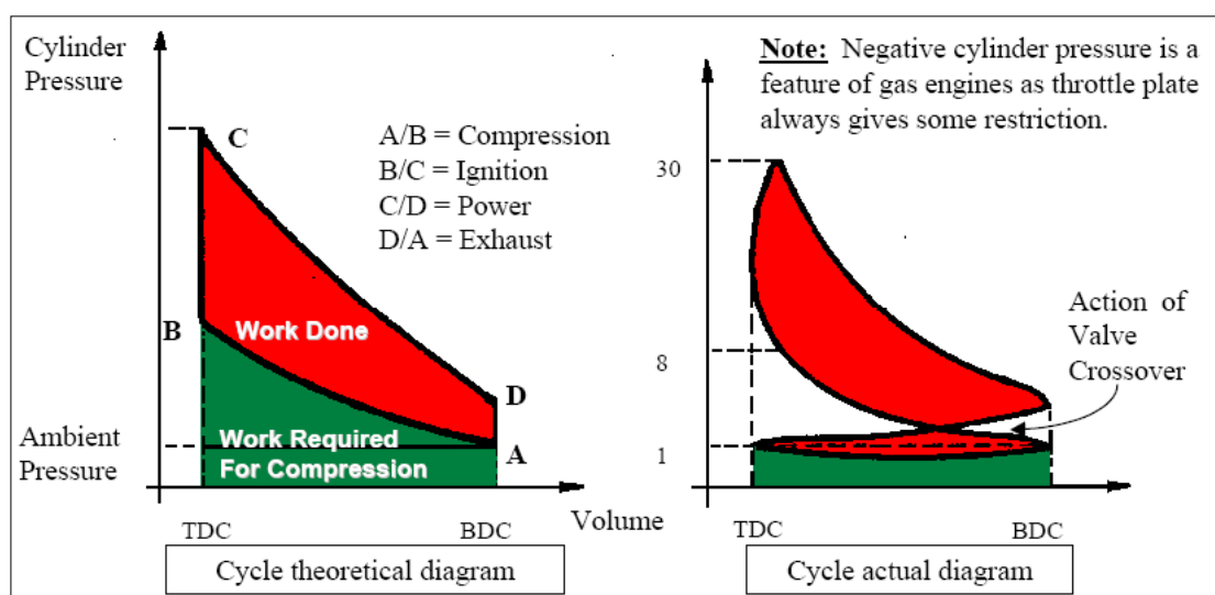
Εικόνα 2.9 Διαγράμματα P-u ιδανικού και πραγματικού κύκλου ΟΤΤΟ
