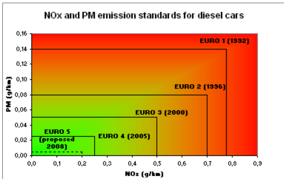
Εικόνα 4.8 Εξέλιξη Ευρωπαϊκών προτύπων και εκπομπές NO x -PM (πετρελαιοκίνητα).
