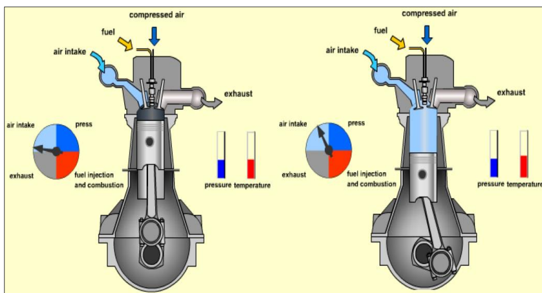
Εικόνα 2.12 Εισαγωγή αέρα στον θάλαμο καύσης (DIESEL-cycle)
