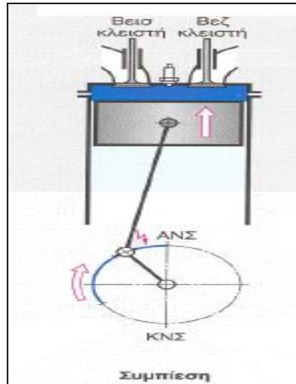
Εικόνα 2.5 Ισεντροπική συμπίεση καύσιμου μίγματος(OTTO-cycle)
