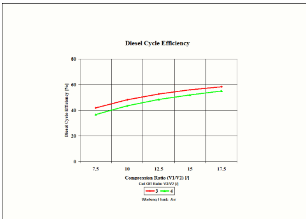
Εικόνα 2.17 Διαγραμματική απεικόνιση συσχέτισης βαθμού απόδοσης με τον λόγο συμπίεσης και λόγο αποκοπής (κύκλος DIESEL).
