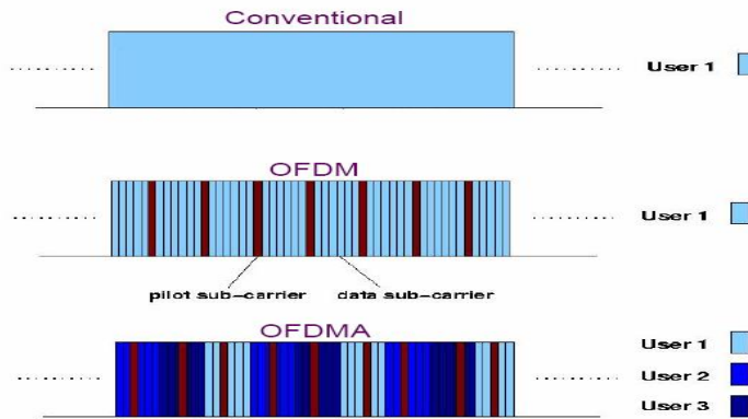
Εικόνα 23 : OFDM διαχωρισμός υπο-καναλιών (sub-channels) [26]
