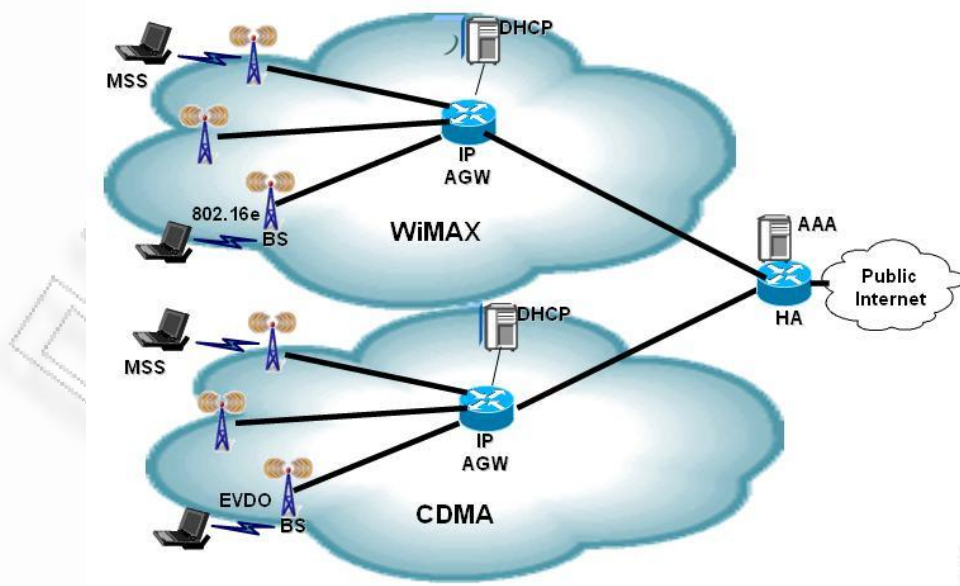
Εικόνα18 : Συστατικά ενός δικτύου WiMAX[67]
