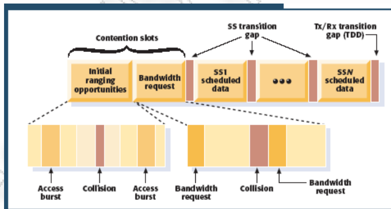
Εικόνα22: Διαδικασία στρώματος MAC [25]
