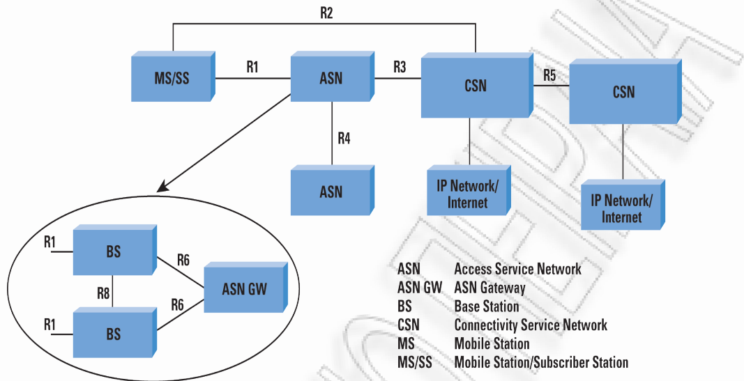
Εικόνα 17 : Αρχιτεκτονική ενός δικτύου WiMAX με τα λειτουργικά τμήματα και τα σημεία διασύνδεσης [68]
