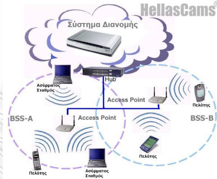
Εικόνα 4 : Δομημένη τοπολογία ασύρματου δικτύου [8]
