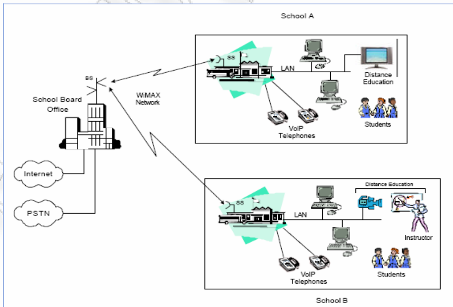
Εικόνα 34 :ΕκπαιδευτικάΔίκτυα[40]
