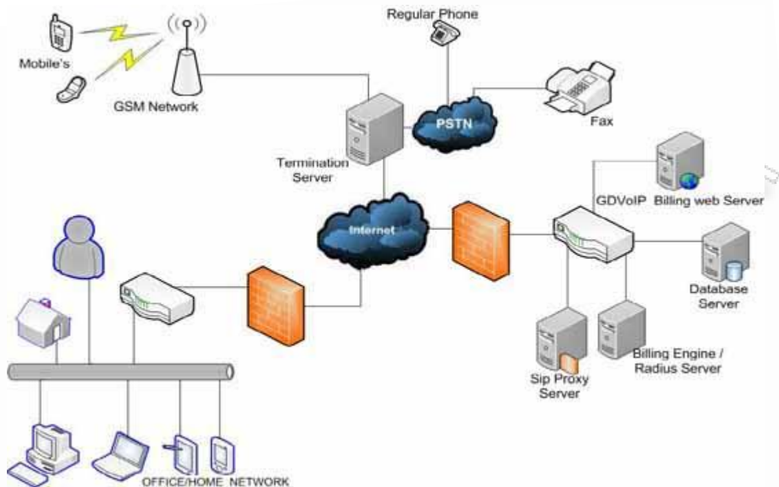
Εικόνα 16: Αρχιτεκτονική Asterix (www.openvoips.com)
