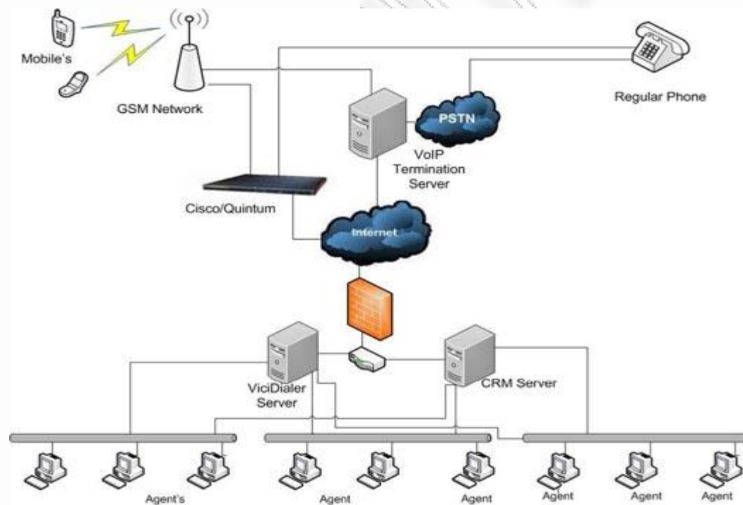
Εικόνα 18 : Αρχιτεκτονική πλευρά vicidial
