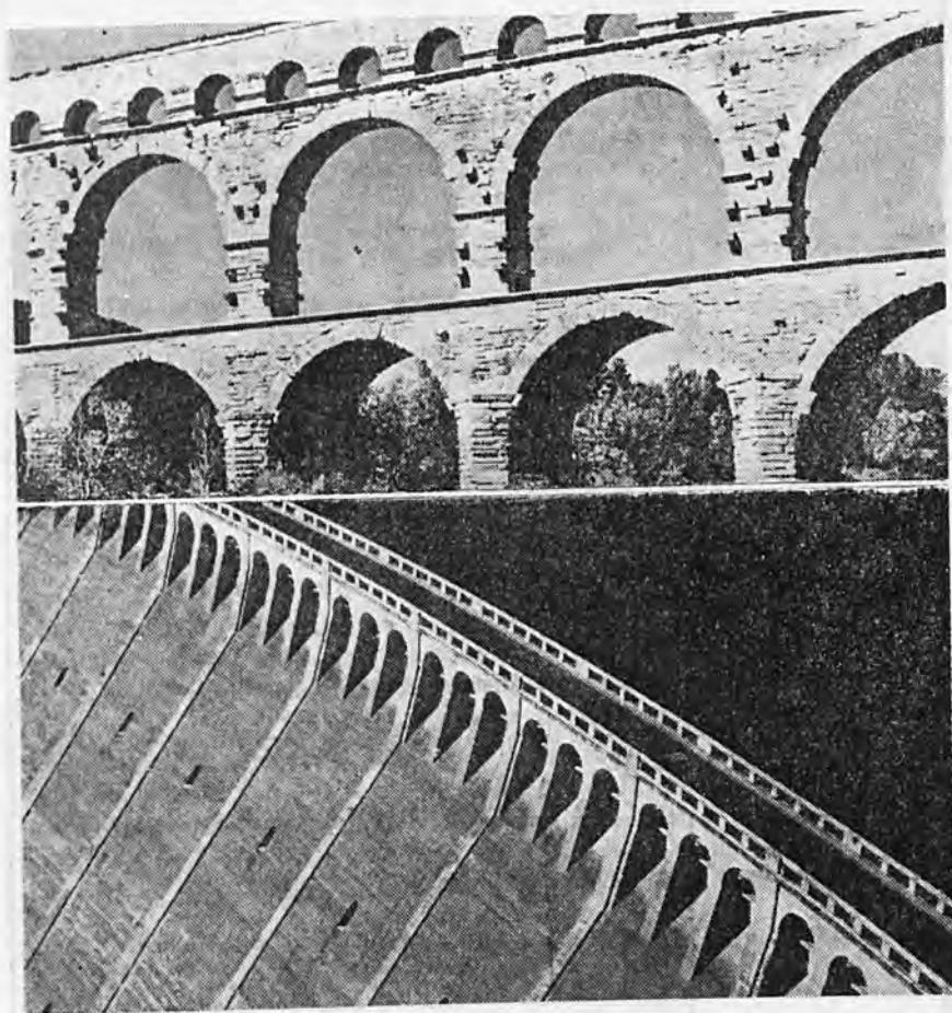
Ἄλλοις καὶ τῶρα Ἄνω: Γέφυρα τοῦ 1ου π.Χ. αἰῶνος — Κάτω: Τροάσιον φράγμα.
